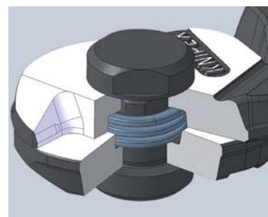
Verzonken openingsveer
