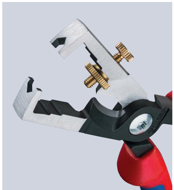
Längenmarkierung: Profilierung der Innenseite unterstützt beim wiederholten Abisolieren gängiger Längen (11 mm und 16 mm)
