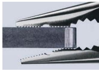
Spitz-Kombizange: ideal zum Greifen flacher Teile dank einseitig konvexer Greiffläche
